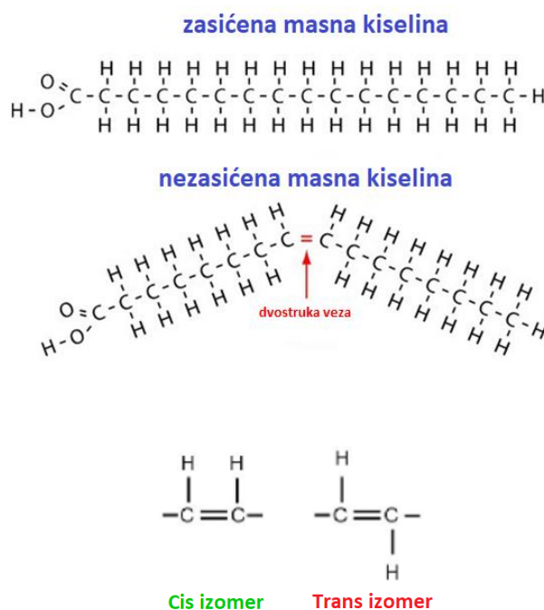
Slika 1. Strukturna formula zasićenih i nezasićenih masnih kiselina, te cis i trans konformacija
