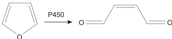
Slika 6. – Nastanak cis -2-buten-1,4-diala iz furana
