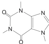
Slika BTox14 – Strukturna formula kofeina, najpoznatijeg ksantina
