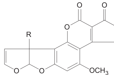
Slika 4. Strukturna formula aflatoksina B1 i M1
